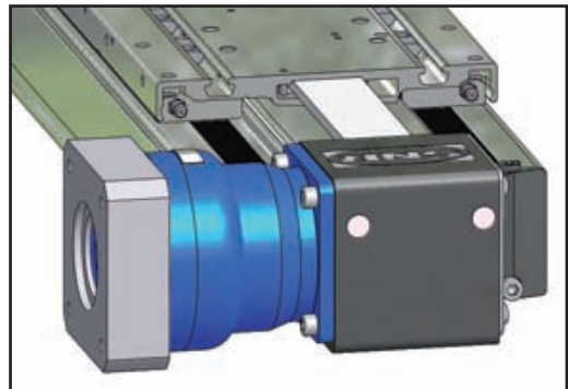
Baureihe AXDL_Z
