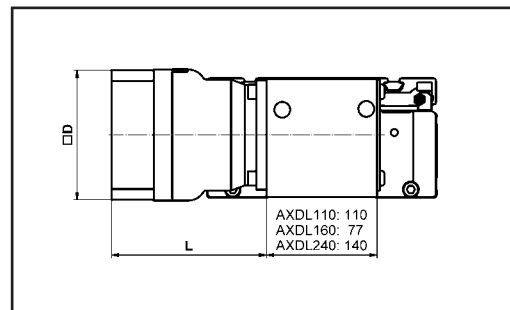
Baureihe AXDL_Z
