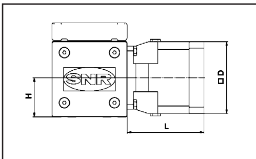
Baureihe AXC_Z
