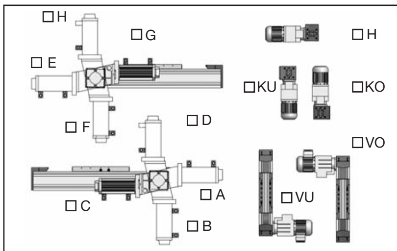
Anbaulage Winkelgetriebe
