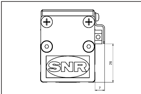
Anbauvariante 3
