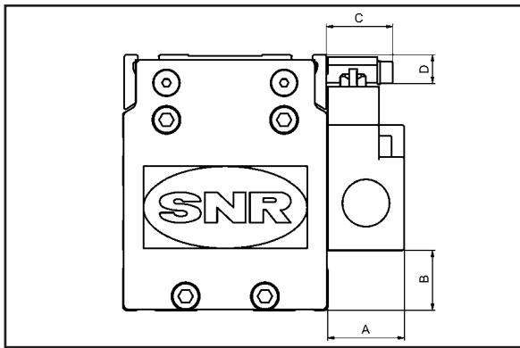
Anbauvariante 1
