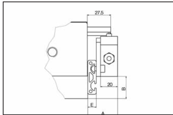
Anbauvariante 2
