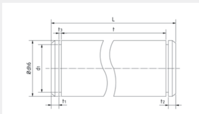
Gorge pour segment d'arrêt selon DIN 471
