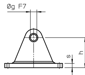
2 Lagerfüße
