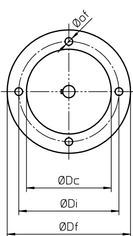
Antriebsgetriebemotor - Anbau
