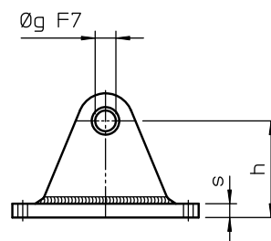
2 Lagerfüße
