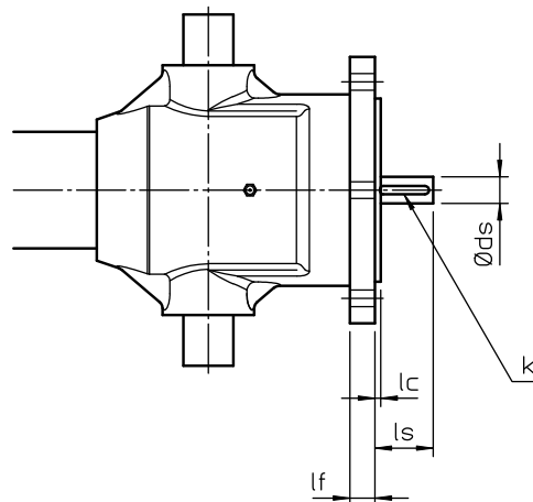
Antriebsgetriebemotor - Anbau
