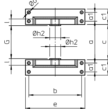
2 Lagerfüße
