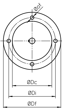
Antriebsgetriebemotor - Anbau
