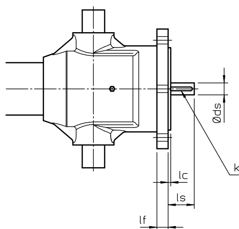
Antriebsgetriebemotor - Anbau
